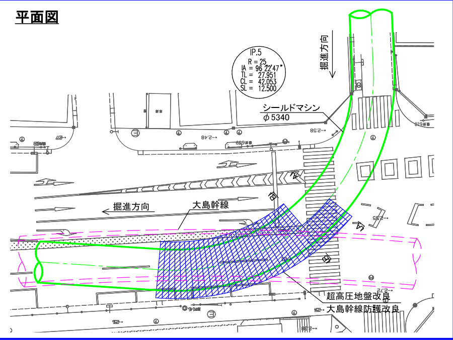
図－2 既設大島幹線防護改良概要図
