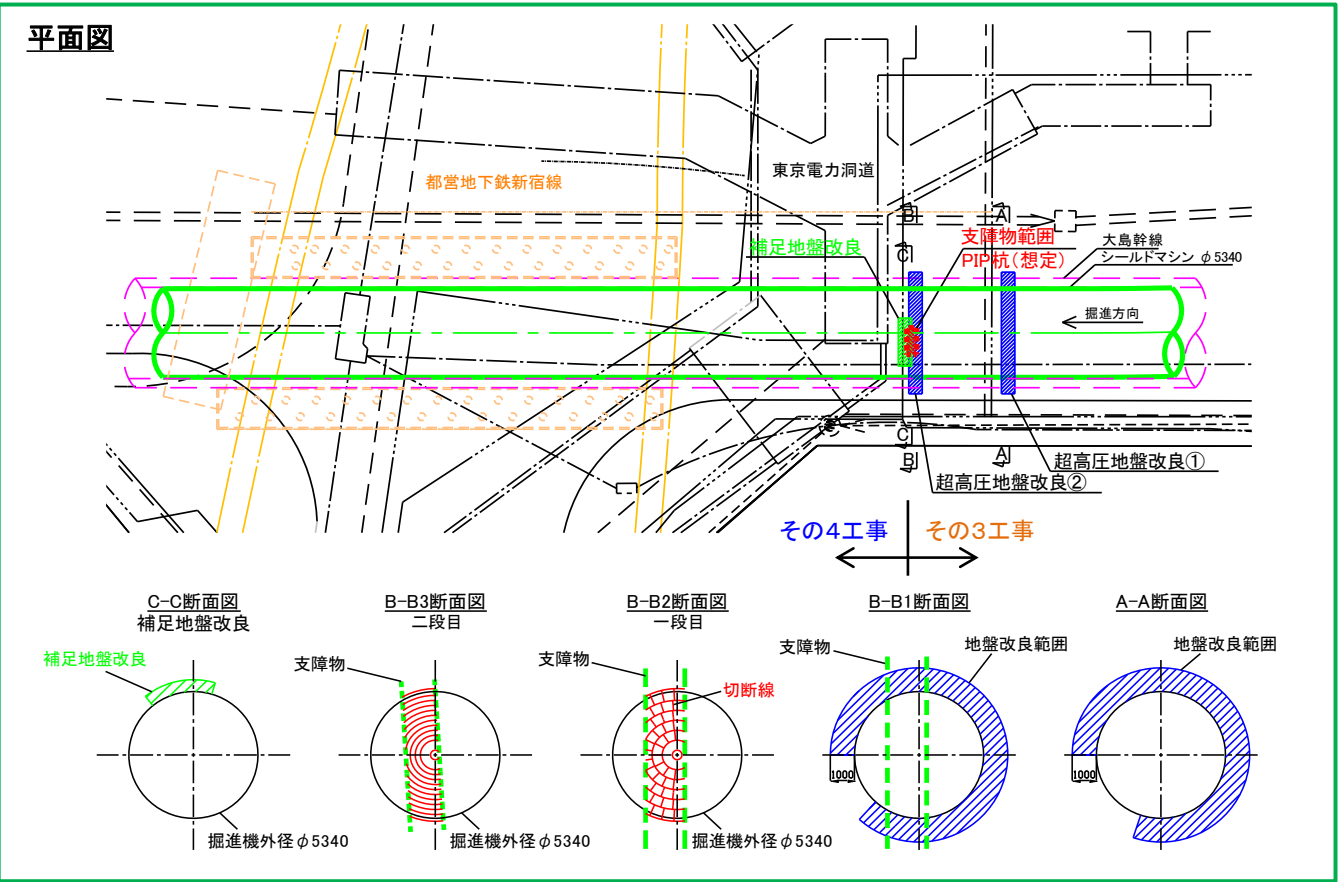
図－4 支障物切断改良概要図
