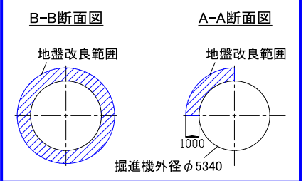
図－3 改良断面図
